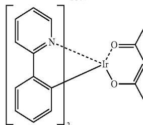
Ir(ppy) 2 (acac)
