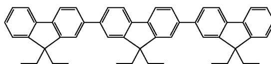
E3
