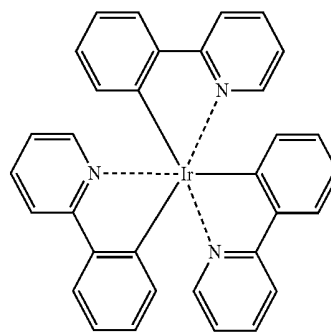
Ir(ppy) 3
