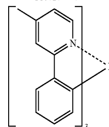
Ir(mpyp) 3
